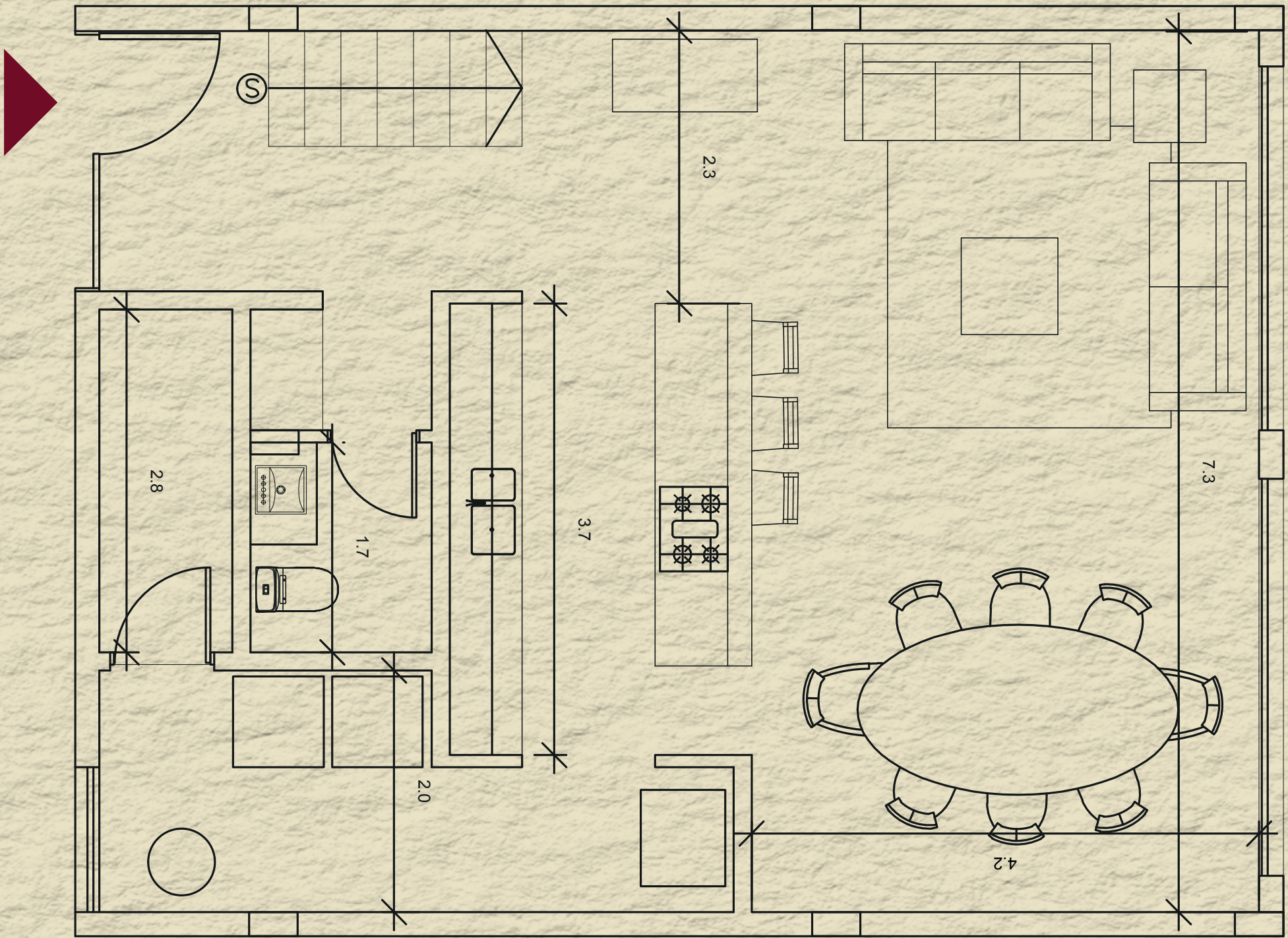
PLANTA BAJA
